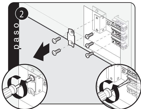
Retire el soporte de alivio de tensión del cable de alimentación y los tres tornillos de montaje del cable de alimentación en el bloque de terminales.
