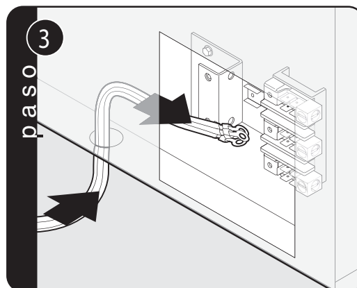
Pase el cable de alimentación a través del agujero en la parte inferior de la parte de atrás de la estufa.
