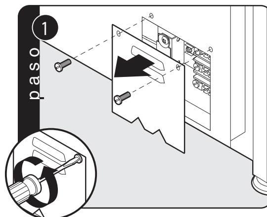
Retire la puerta de acceso.
