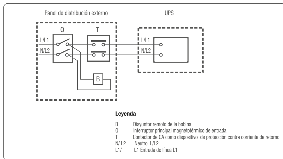
Diagrama 1: Cableado para el protector de corriente de retorno externo
