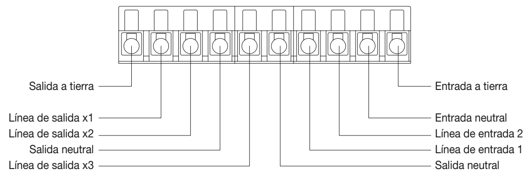
Diagrama de cableado del bloque de terminales de la UPS
