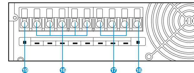
Diagrama 3: Terminales de entrada y salida del transformador de aislamiento
